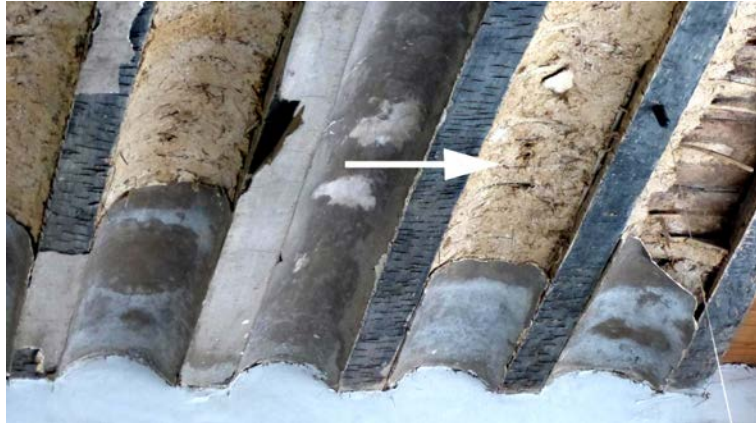
Illustration 2: Languettes ou voussettes vues par dessous. (Marie-Christine Geib-Munier)
