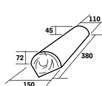
A000 3810 * About d'arêtier de chevauchement tige de botte
