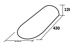
A000 1420 * About de fatière demi-ronde
