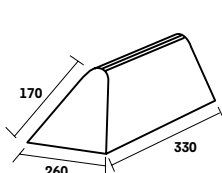
A000 1810 * About de fatière angulaire
