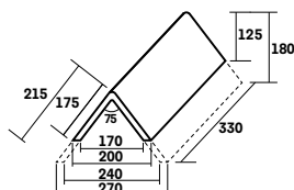
A000 1870 - A000 1880 * Fatière angulaire 75 pour forte pente 3,0 au ml
