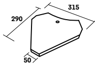
A000 3970 * Tuile de noue pour 16 x 27 10,0 au ml
