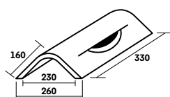
A000 1280 * Fatière Patrimoine de ventilation 36 cm 3,0 au ml
