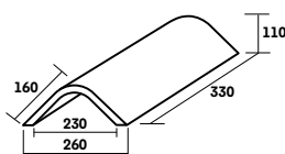
A000 1200 * Fatière Patrimoine 3,0 au ml
