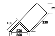
A000 1800 * Fatière angulaire 90 3,0 au ml
