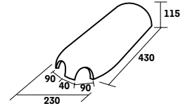
A000 5880 Rencontre fatière demi-ronde 2 pans
