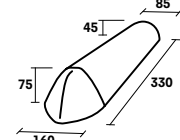
A000 3910 * About d'arêtier Patrimoine
