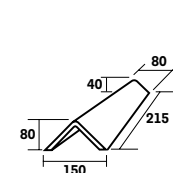
A000 3700 * Cornier 10,0 au ml
