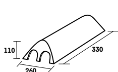
A000 5890 * Rencontre fatière Patrimoine 2 pans
