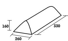
A000 1220 * About de fatière Patrimoine
