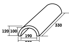
A000 1400 * Fatière demi-ronde 3,0 au ml
