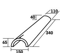
A000 3800 * Arêtier de chevauchement tige de botte 3,5 au ml
