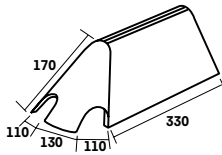
A000 5800 * Rencontre fatière angulaire 2 pans
